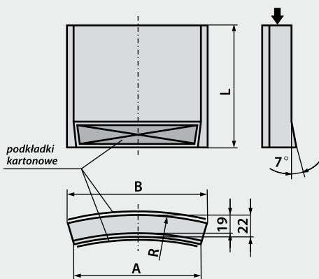
3123 - B / A x L - R...
