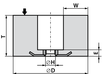
Ściernica garnkowa walcowa z wkładką gwintową 6003 - D × T × H - W...E...
